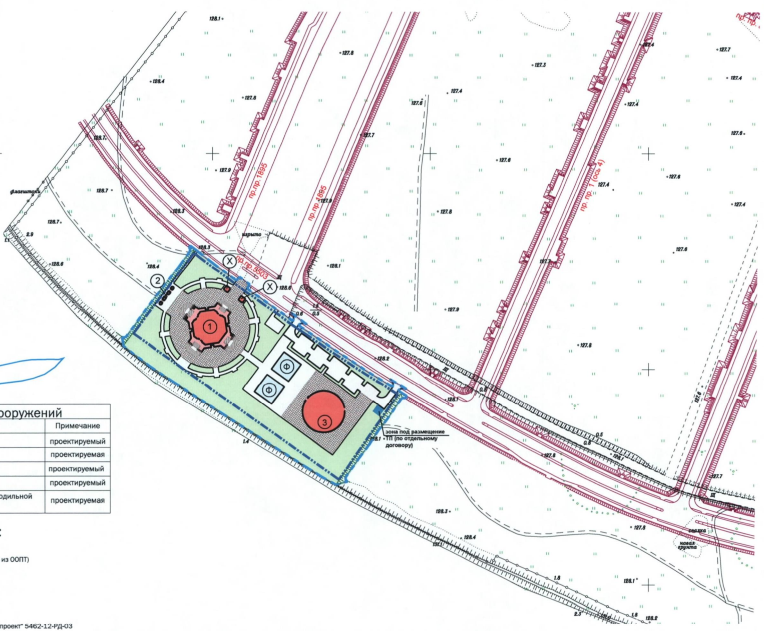
Схема размещения объекта в границах участка по ГПЗУ №RU77179000-046366
